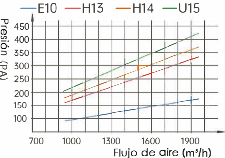
Diagrama de flujo de aire y resistencia 610*610*69
